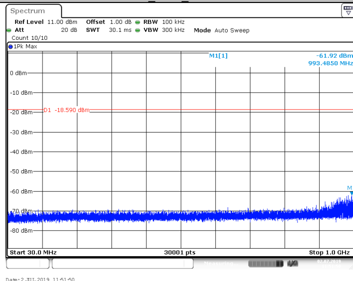
BLE_2402_1000~26500
