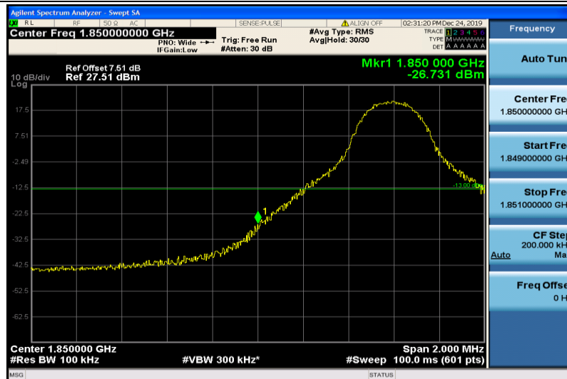
Band2-10MHz-QPSK-18650-1RB#0
