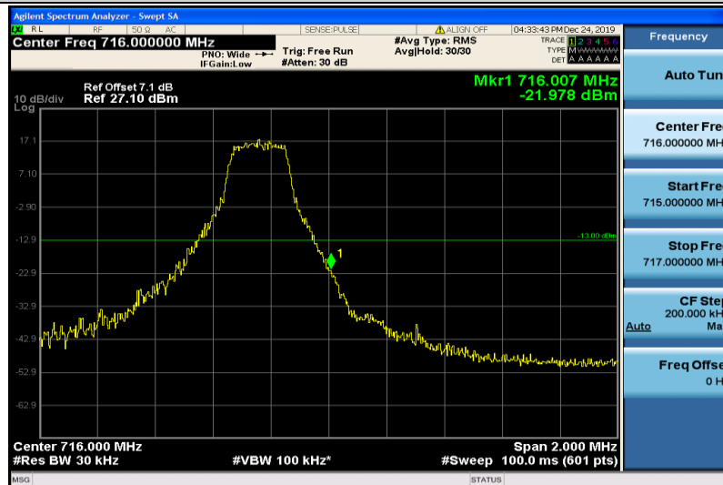
Band12-3MHz-QPSK-23165-1RB#14
