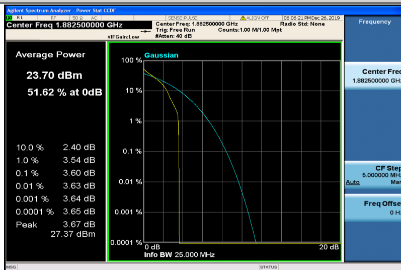
Band25-20MHz-QPSK-26365-1RB#0
