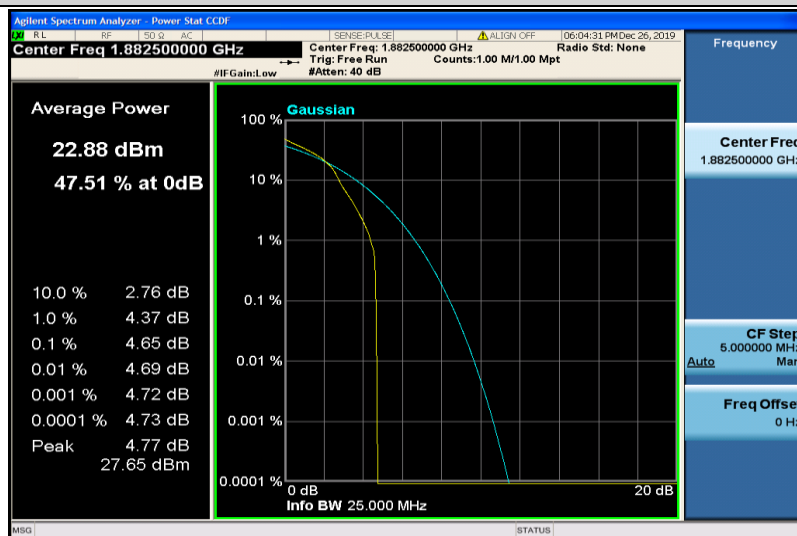
Band25-10MHz-16QAM-26365-1RB#0
