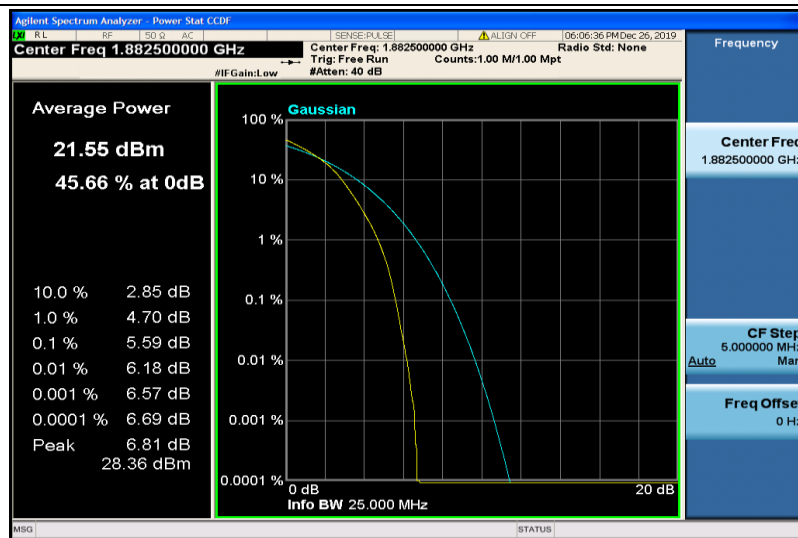
Band25-20MHz-16QAM-26365-100RB#0
