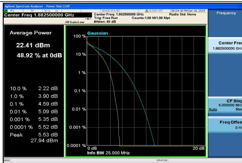
Band25-10MHz-QPSK-26365-50RB#0
