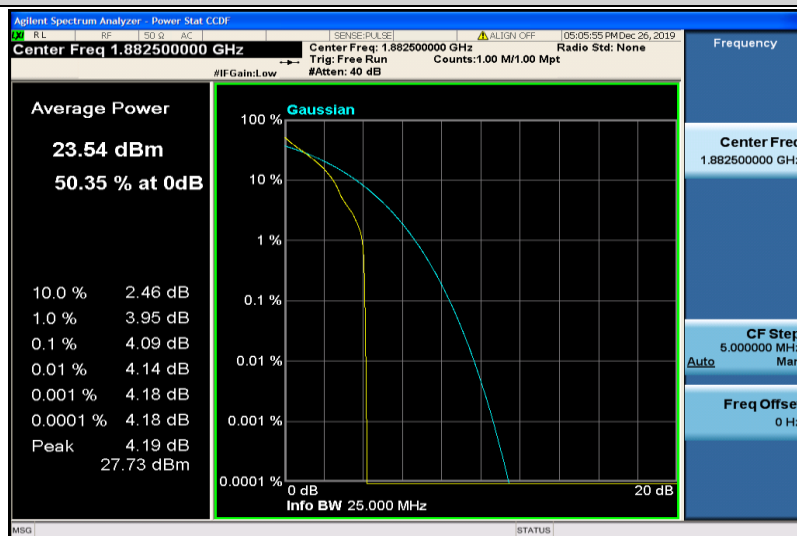
Band25-3MHz-QPSK-26365-1RB#0
