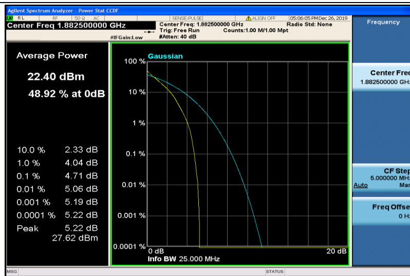
Band25-3MHz-QPSK-26365-15RB#0
