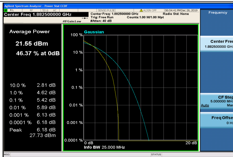
Band25-10MHz-16QAM-26365-50RB#0
