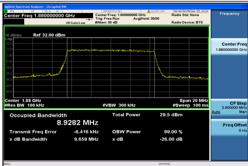
Band2-10MHz-16QAM-18900-50RB#0-8.9282
