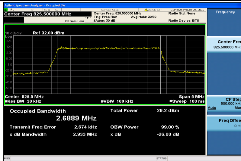
Band5-3MHz-QPSK-20415-15RB#0-2.6889
