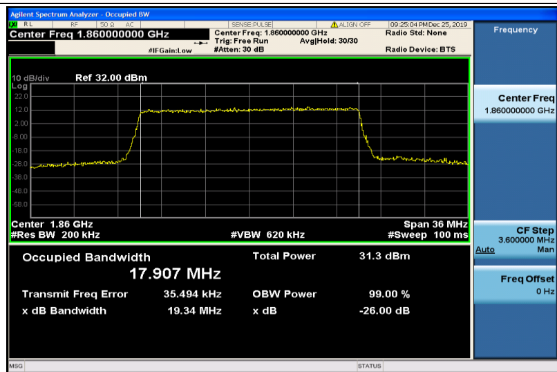
Band2-20MHz-QPSK-18700-100RB#0-17.907
