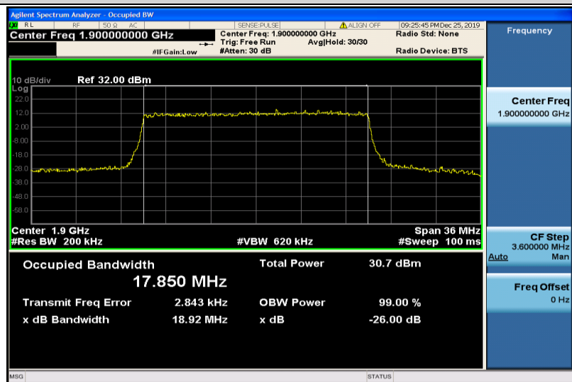
Band2-20MHz-QPSK-19100-100RB#0-17.850
