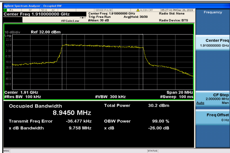
Band25-10MHz-QPSK-26640-50RB#0-8.9450
