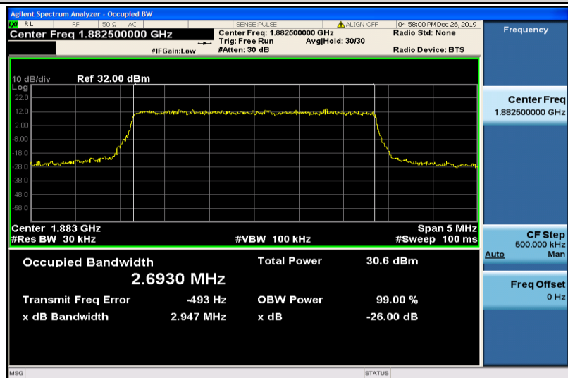
Band25-3MHz-QPSK-26365-15RB#0-2.6930
