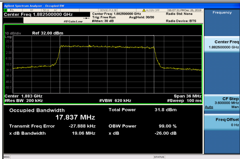
Band25-20MHz-QPSK-26365-100RB#0-17.837
