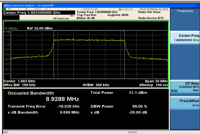
Band25-10MHz-QPSK-26365-50RB#0-8.9288
