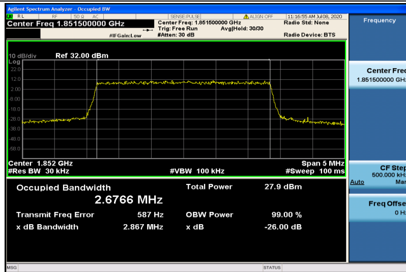
Band2-3MHz-QPSK-18615-15RB#0-2.6766
