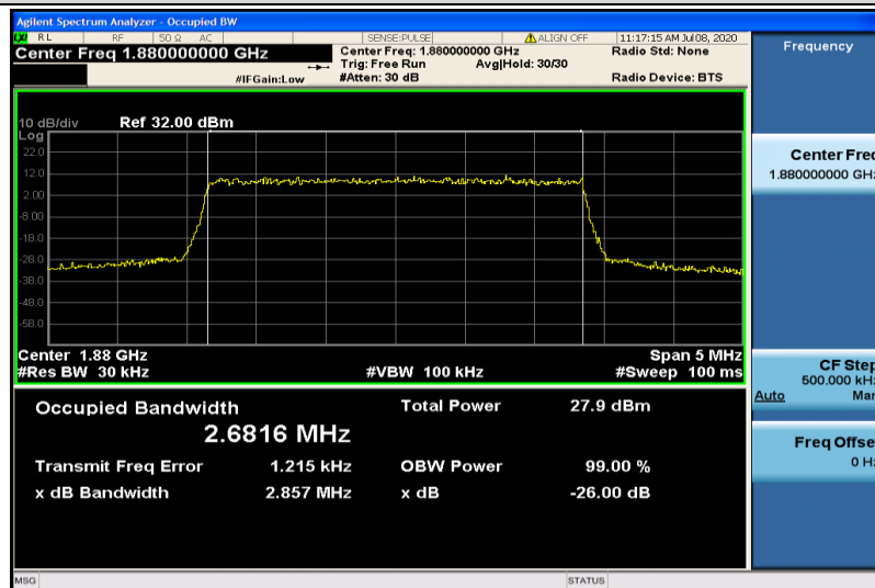
Band2-3MHz-QPSK-18900-15RB#0-2.6816
