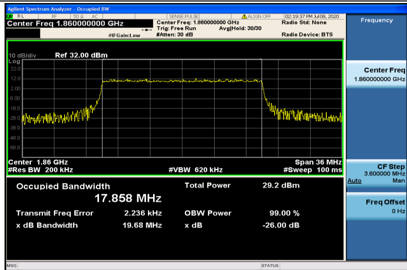
Band2-20MHz-QPSK-18700-100RB#0-17.858
