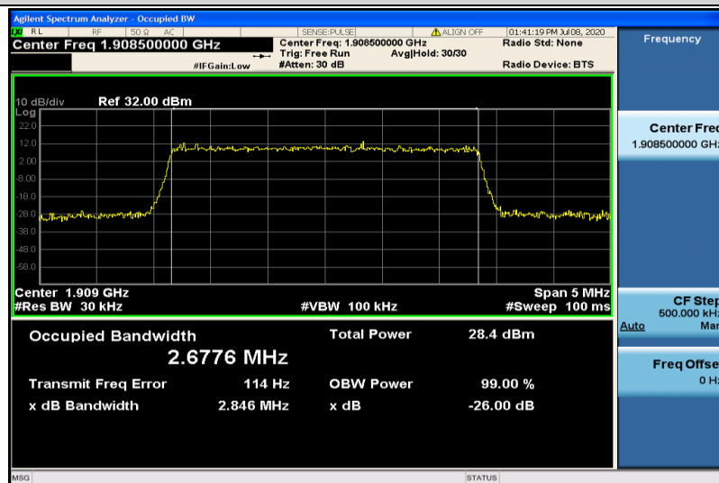
Band2-3MHz-QPSK-19185-15RB#0-2.6776
