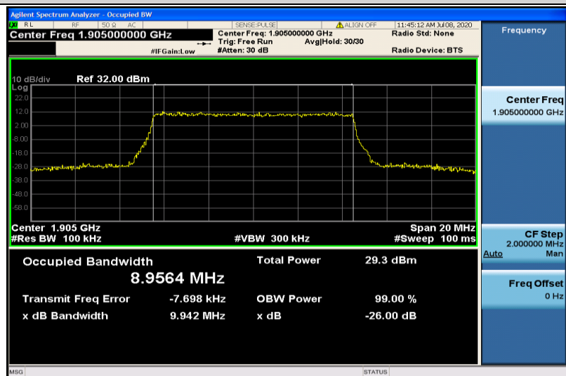
Band2-10MHz-QPSK-19150-50RB#0-8.9564
