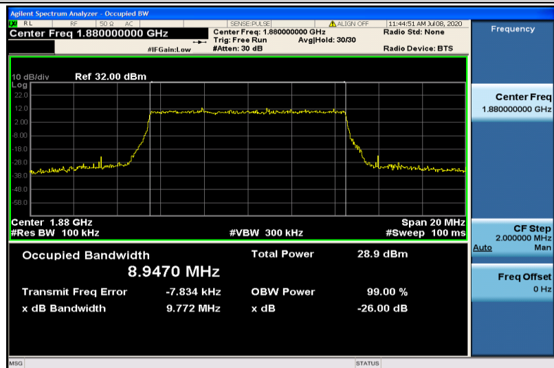
Band2-10MHz-QPSK-18900-50RB#0-8.9470
