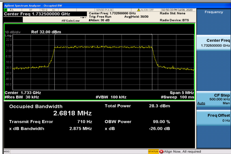
Band4-3MHz-QPSK-20175-15RB#0-2.6818
