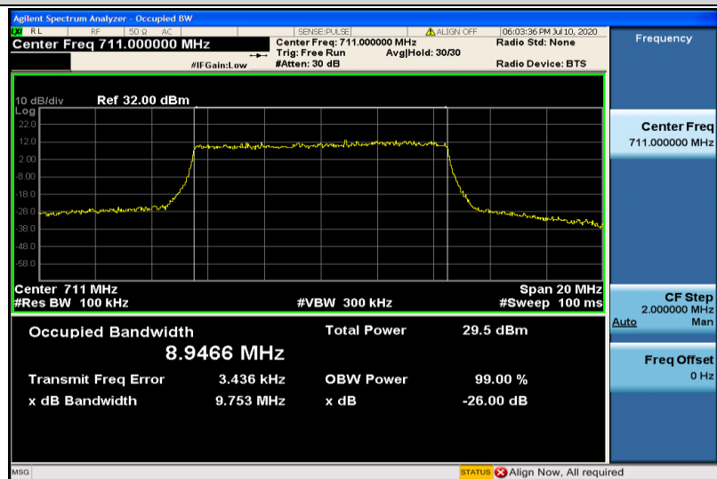
Band12-10MHz-QPSK-23130-50RB#0-8.9466
