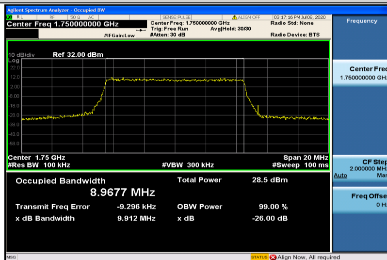
Band4-10MHz-QPSK-20350-50RB#0-8.9677
