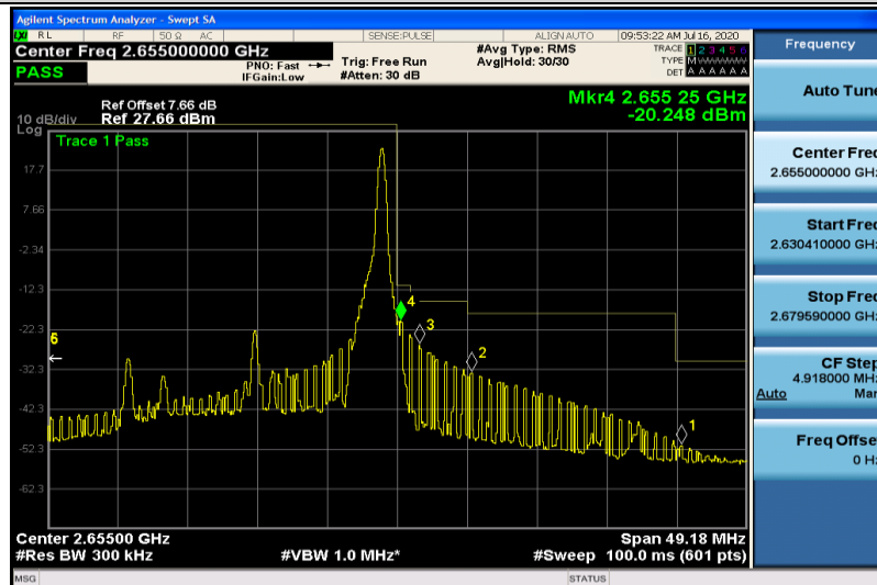
Band41-20MHz-QPSK-41140-1RB#99
