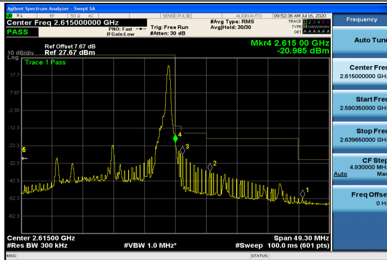
Band41-20MHz-QPSK-40740-1RB#99
