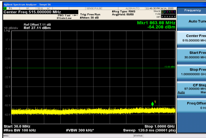
Band25-20MHz-QPSK-26590-1RB#0-30~1000MHz
