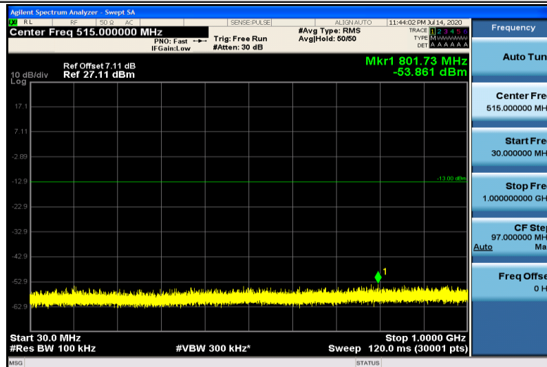
Band25-20MHz-QPSK-26140-1RB#0-30~1000MHz
