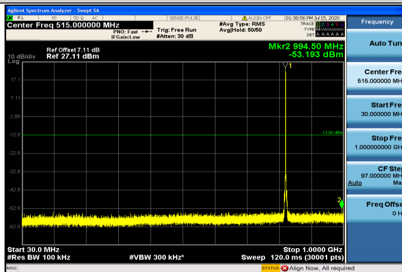
Band26-1.4MHz-QPSK-26797-1RB#0-30~1000MHz
