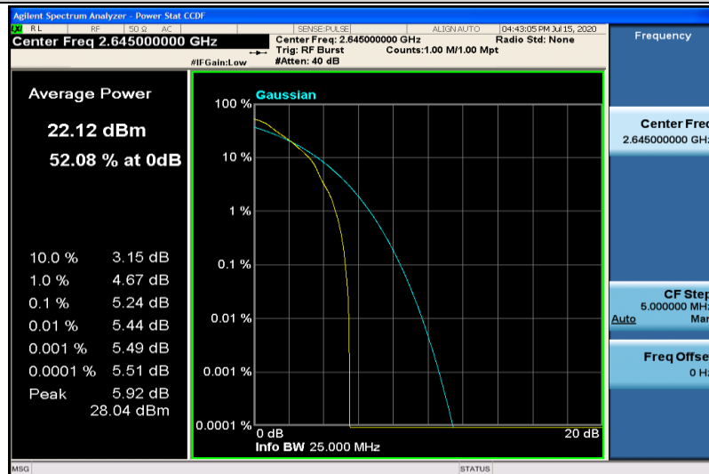
Band41-20MHz-QPSK-41140-1RB#0
