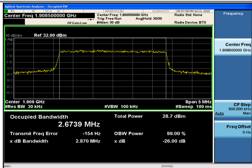
Band2-3MHz-16QAM-19185-15RB#0-2.6739
