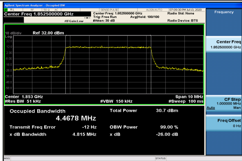
Band2-5MHz-QPSK-18625-25RB#0-4.4678
