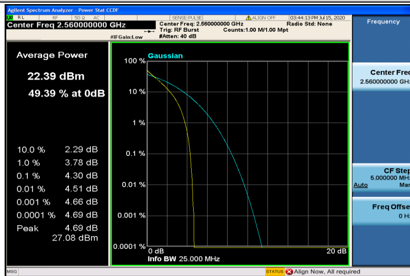
Band41-10MHz-QPSK-40290-1RB#0
