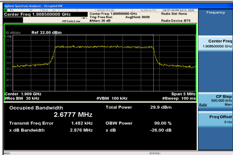
Band2-3MHz-QPSK-19185-15RB#0-2.6777
