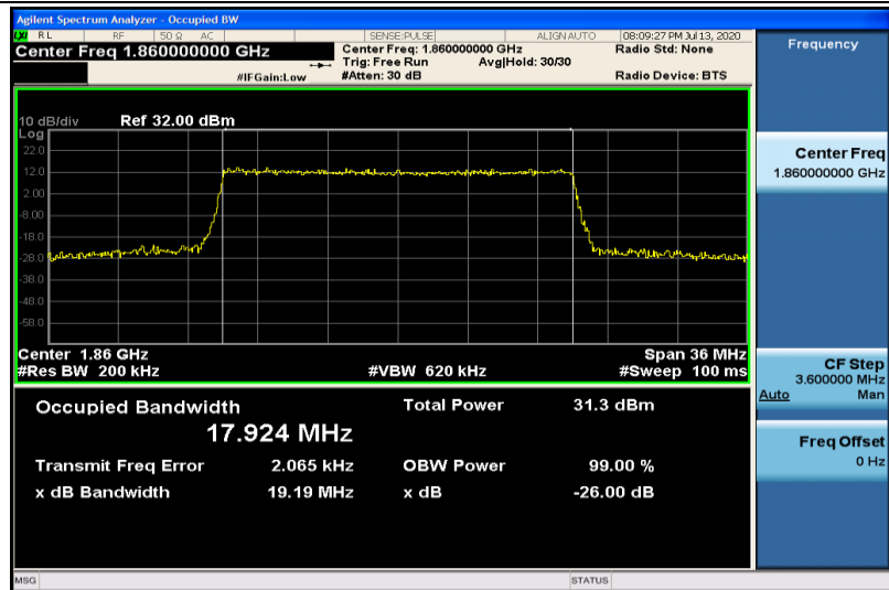
Band2-20MHz-QPSK-18700-100RB#0-17.924
