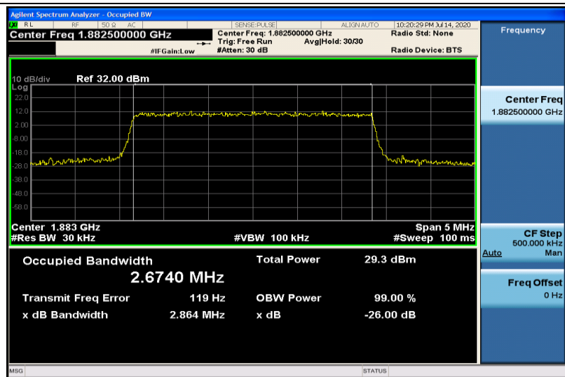
Band25-3MHz-QPSK-26365-15RB#0-2.6740
