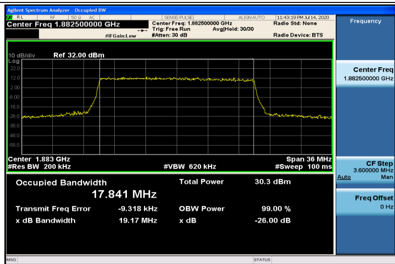
Band25-20MHz-QPSK-26365-100RB#0-17.841
