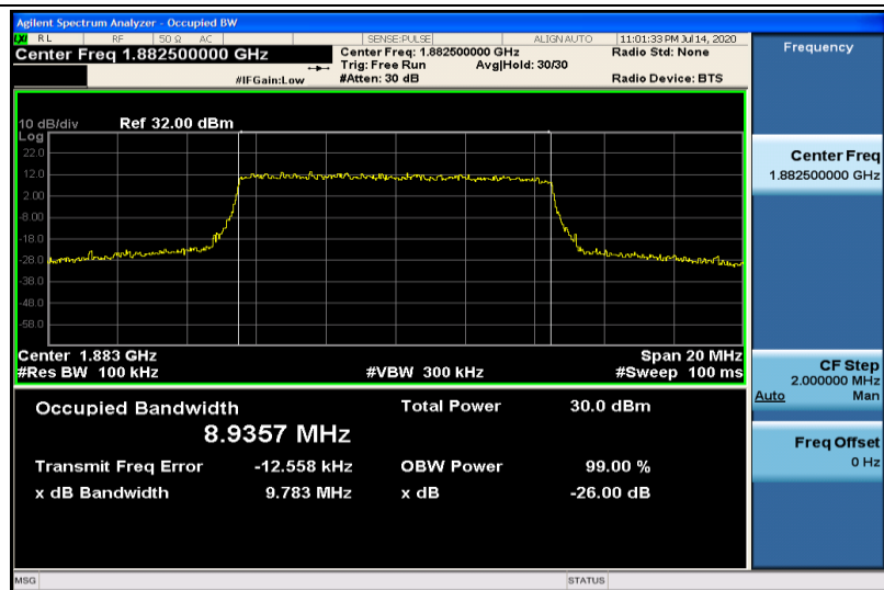
Band25-10MHz-QPSK-26365-50RB#0-8.9357
