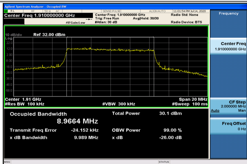
Band25-10MHz-QPSK-26640-50RB#0-8.9664
