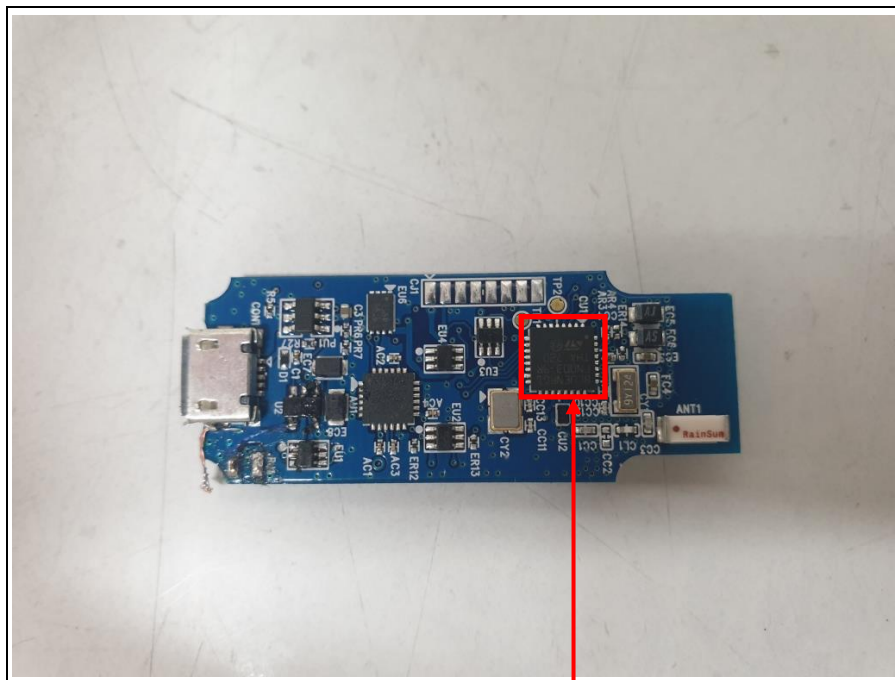
Bluetooth Module
