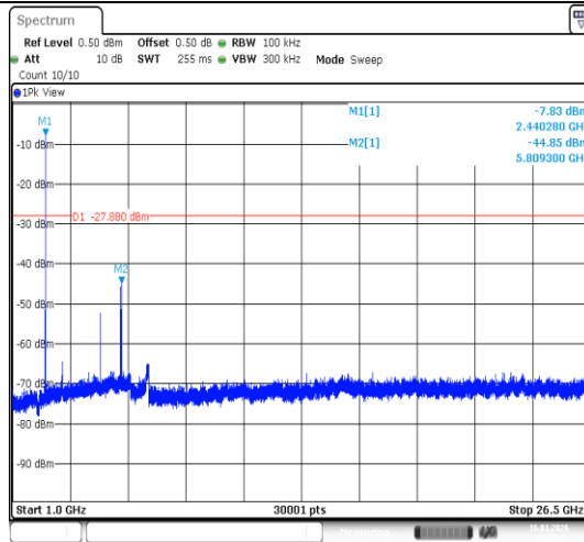
BLE 1M-Ant1-2440-1000~26500-PASS
