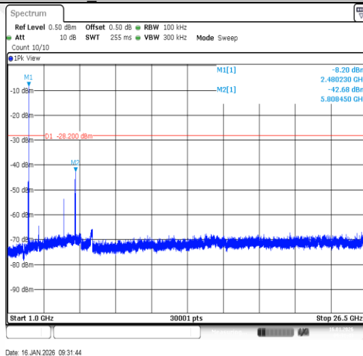
BLE 1M-Ant1-2480-1000~26500-PASS
