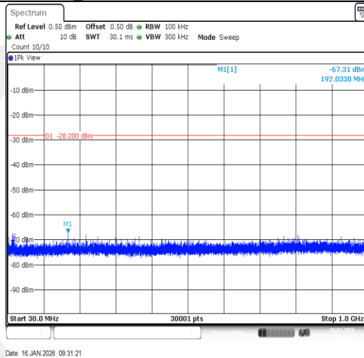
BLE 1M-Ant1-2480-30~1000-PASS
