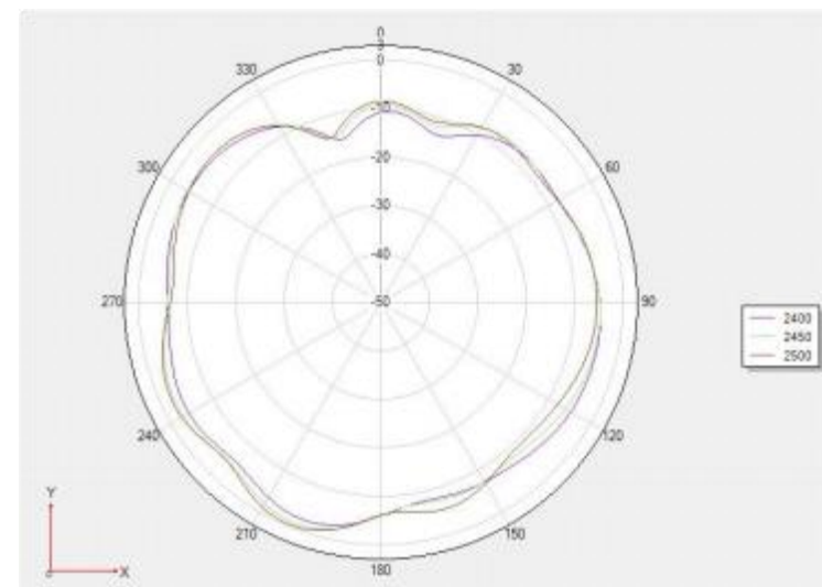
Theta 90 2D图
