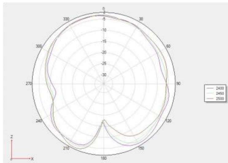
Phi 0 2D图
