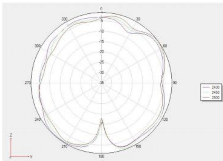
Phi 90 2D图
