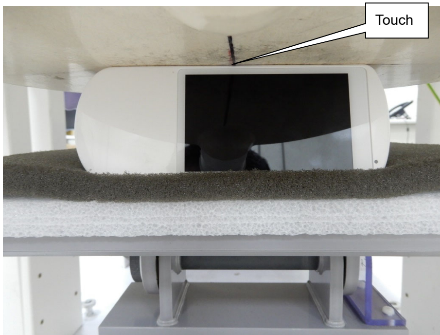
EUT Left-side
