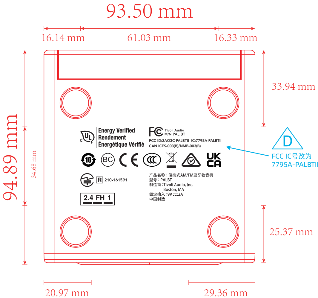
底板丝印图
