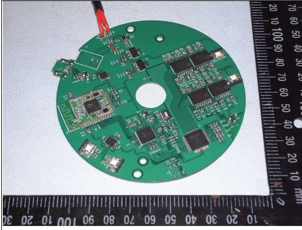
PCB-1
