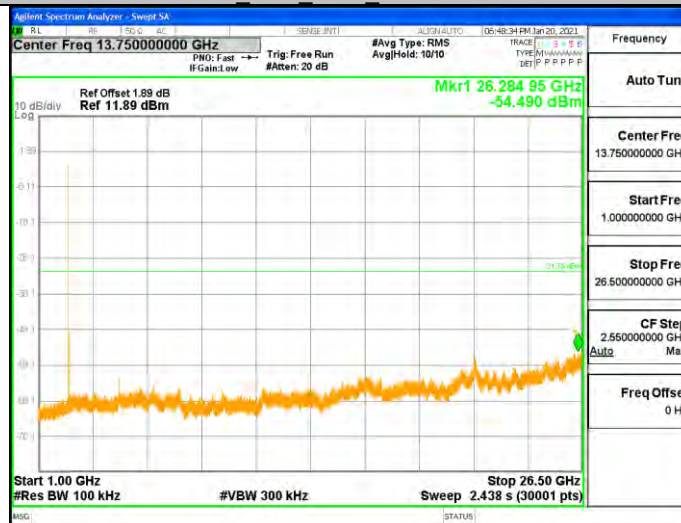
BLE Ant1 2402 1000~26500
