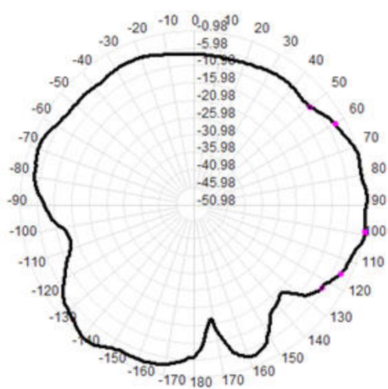
2460.0MHz Total(E1), Max= -0.98dBi
