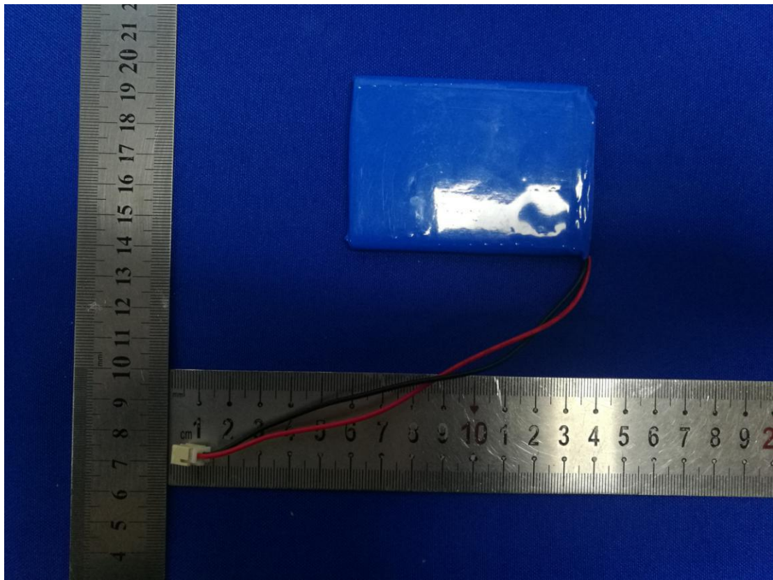
3.7V 4400mAh
