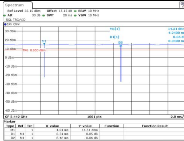
11B_Ant1_2442
