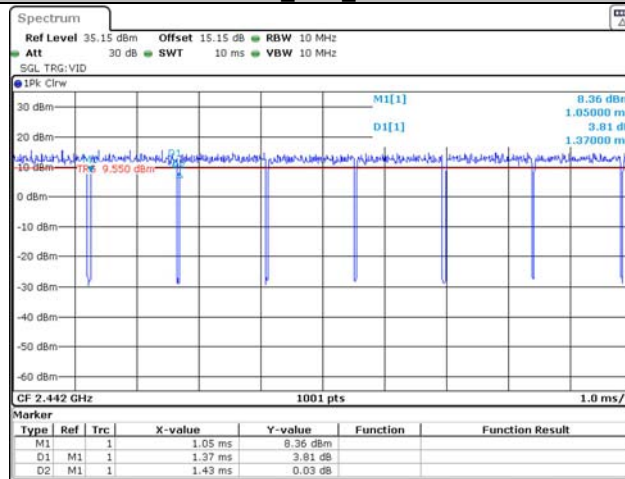
11G_Ant1_2442
