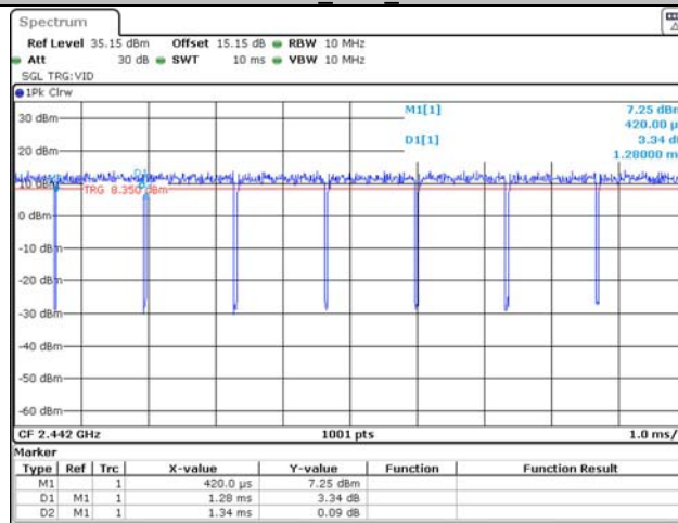
11N20_Ant1_2442
