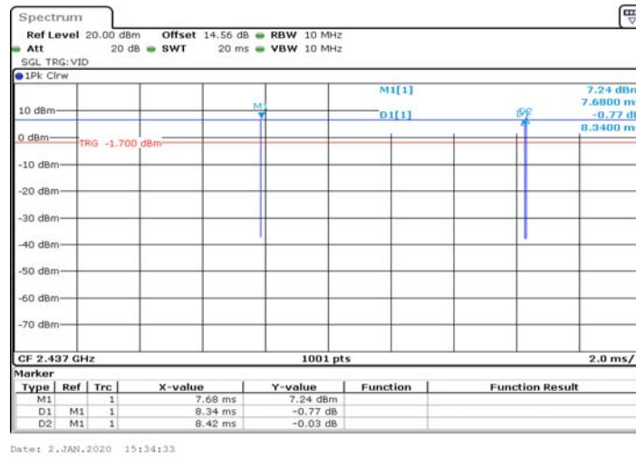
11G_Ant1_2437
