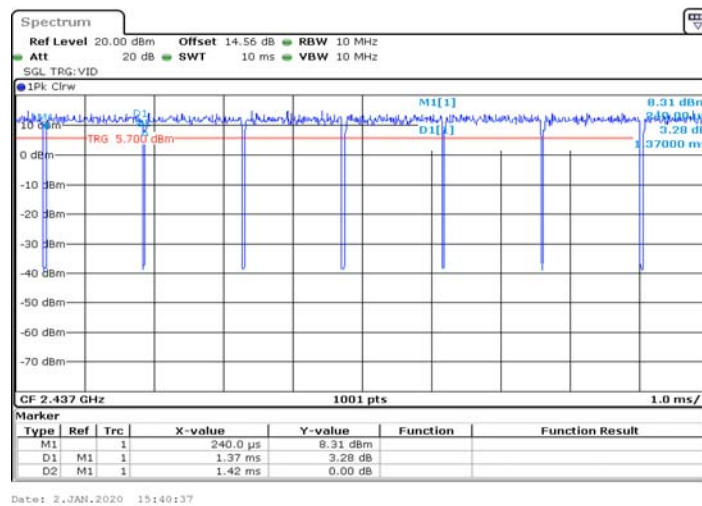
11G_Ant1_2437
