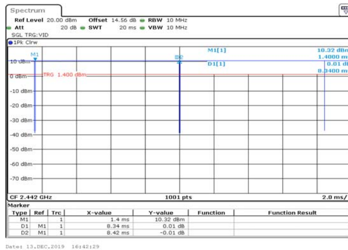
11G_Ant1_2442
