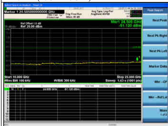
2440MHz(10GHz-25GHz)
