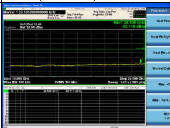
2480MHz(10GHz-25GHz)
