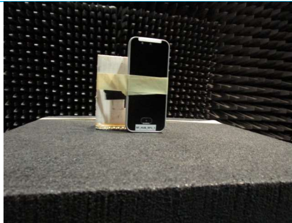
EUT Setup
