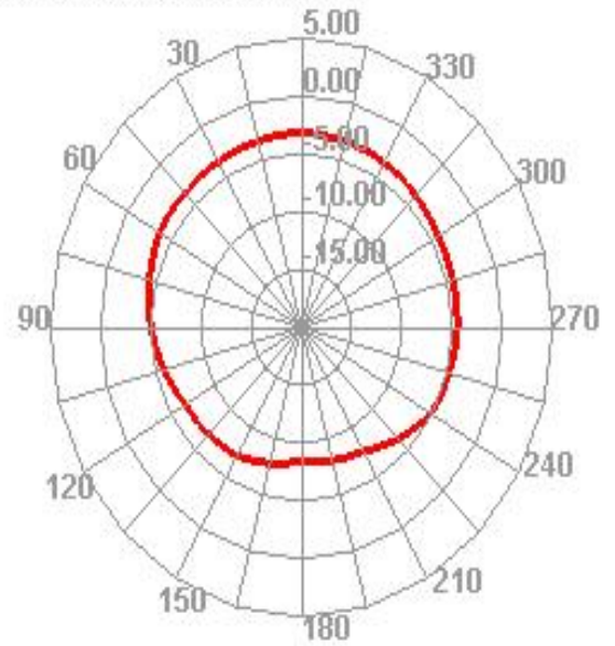
2480.000MHz H
