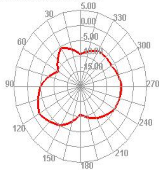
2480.000MHz E2
