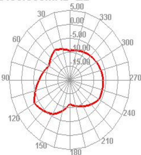
2450.000MHz E2
