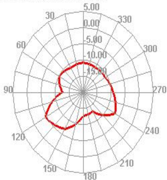
2405.000MHz E2
