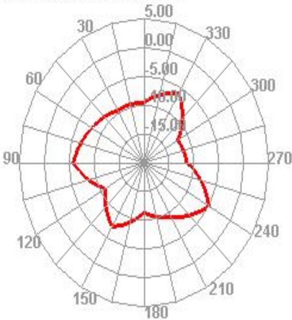
2450.000MHz E1
