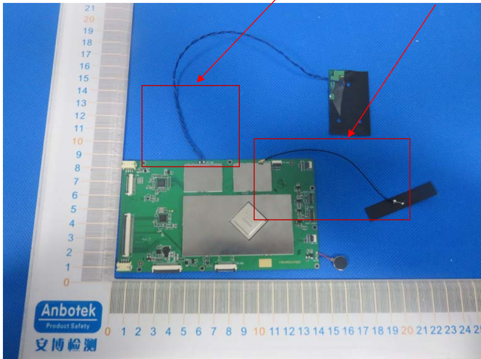
BT&WiFi Antenna
