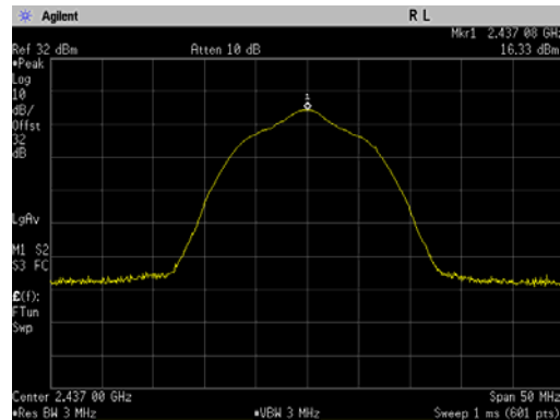
802.11b, 2437 MHz
