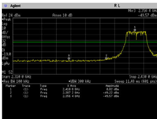
802.11n HT20
