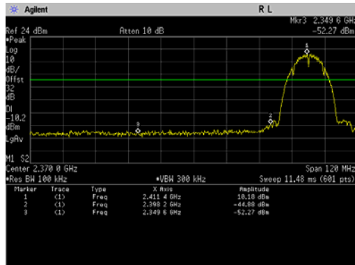
802.11b
