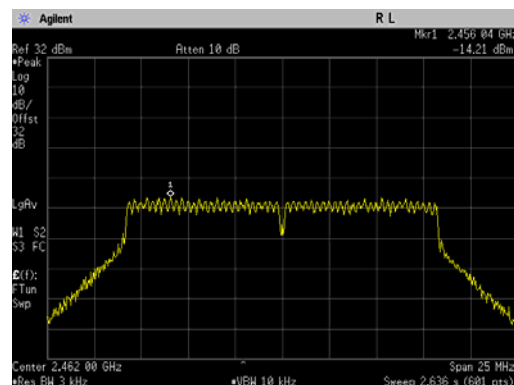
802.11g, 2462 MHz
