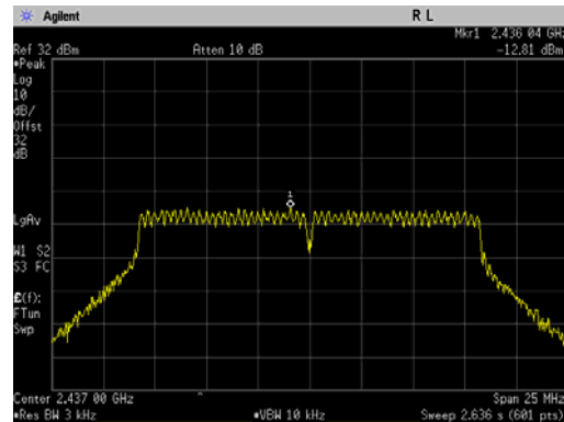
802.11g, 2437 MHz
