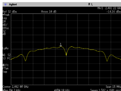
802.11b, 2462 MHz
