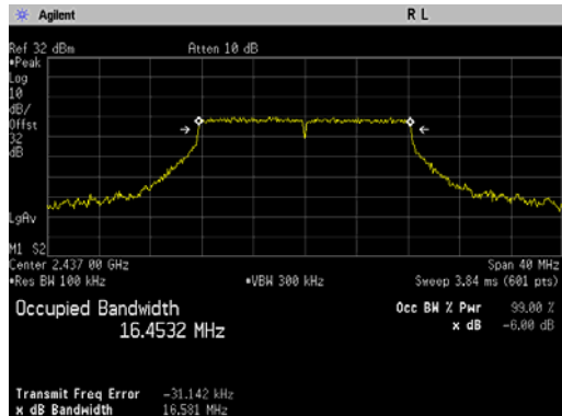
802.11g, 2437 MHz
