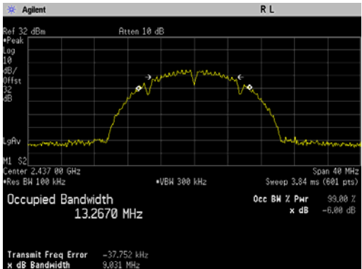
802.11b, 2437 MHz
