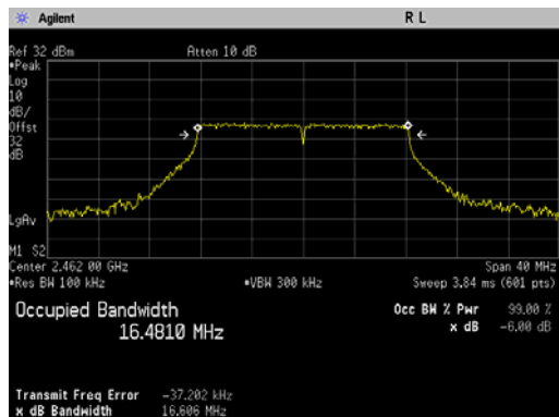
802.11g, 2462 MHz
