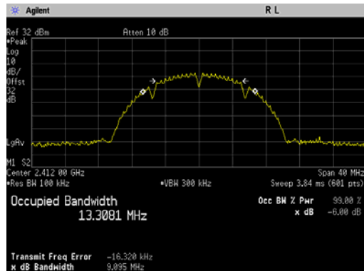
802.11b, 2412 MHz
