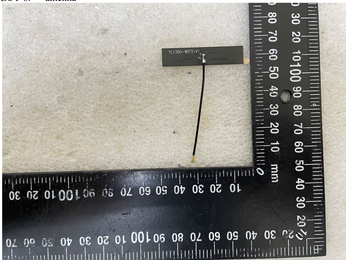
EUT-8. antenna
