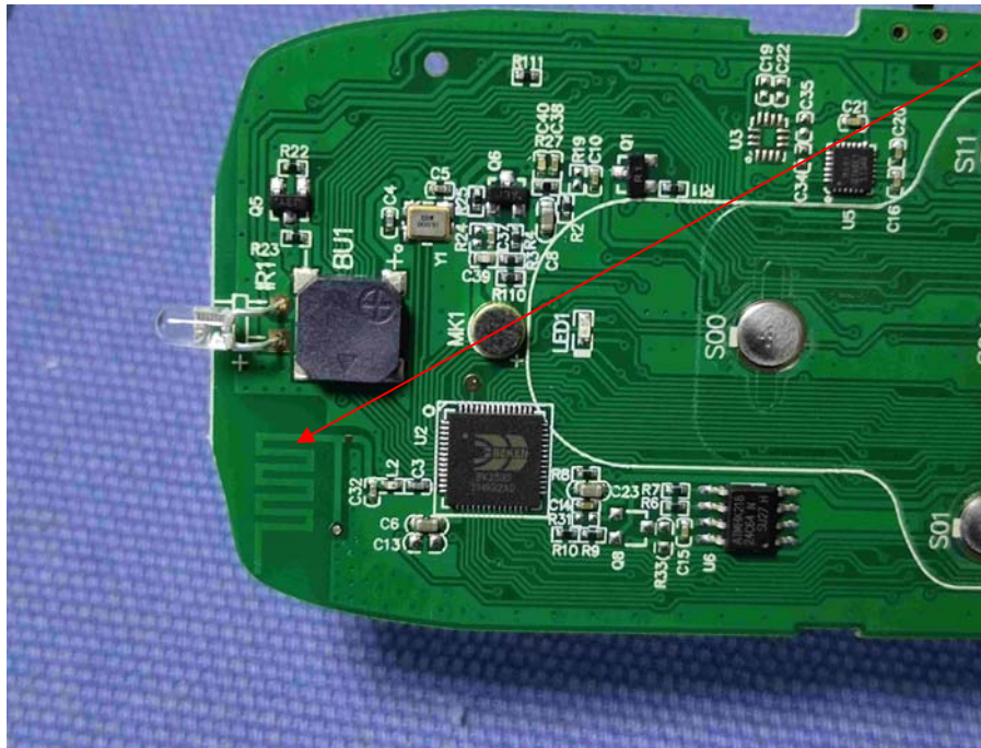
2.4G Antenna
