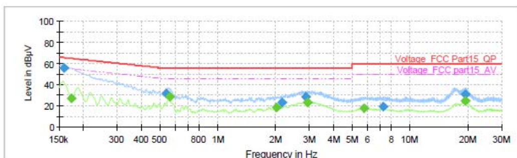
L Line 0.15-30MHz
