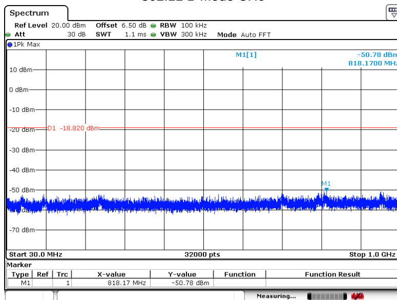
802.11 B Mode CH0
