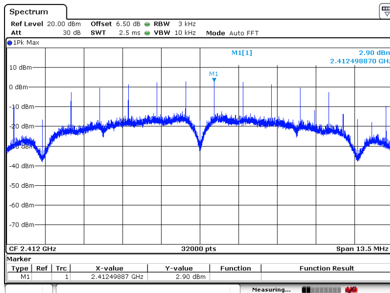
802.11 B Mode CH1
