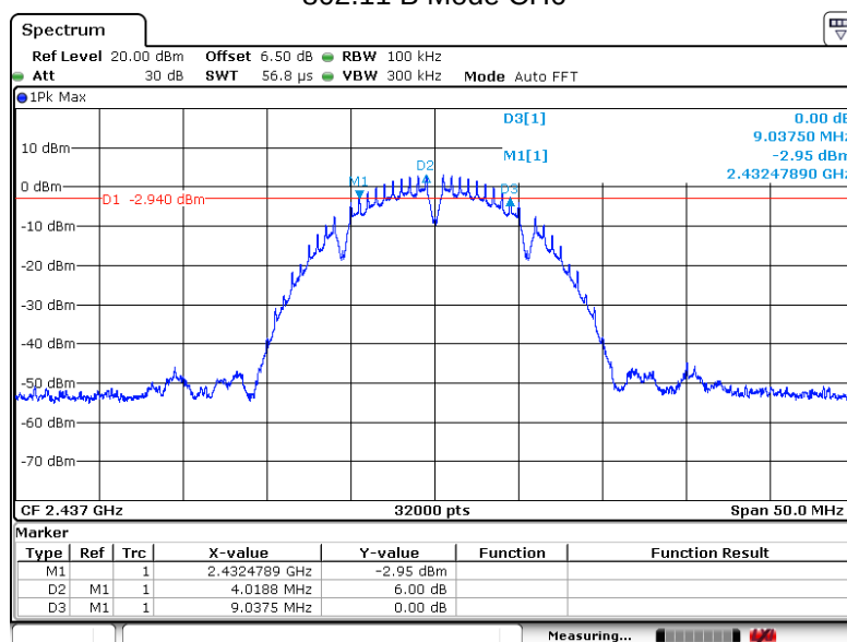
802.11 B Mode CH6
