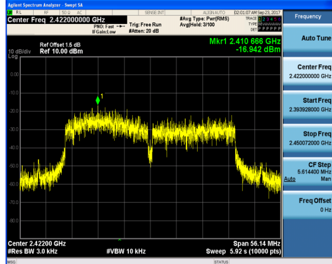
802.11n(HT40)
