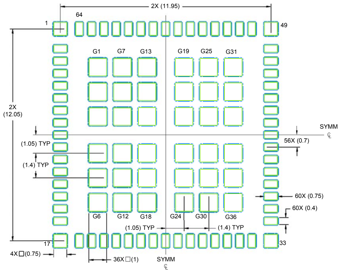
LAND PATTERN EXAMPLE SCALE: 8X
