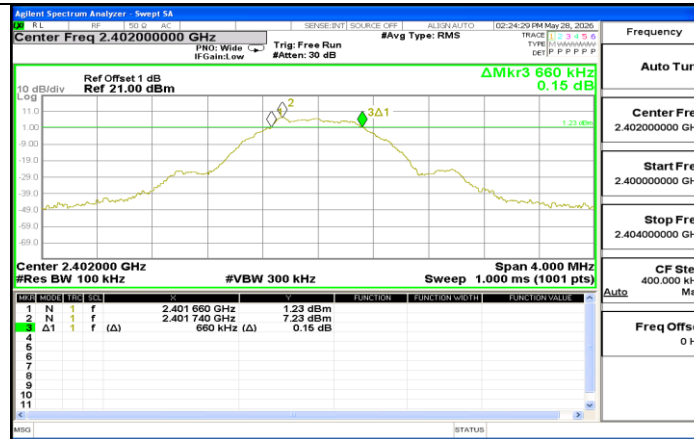
BLE 500K Ant1 2402
