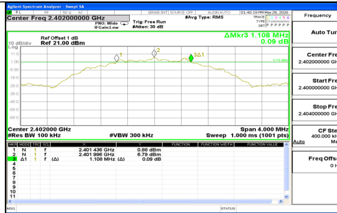
BLE_2M_Ant1_2402
