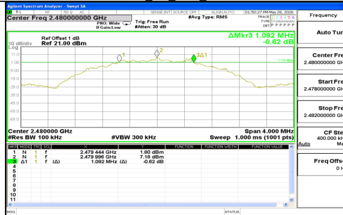
BLE_2M_Ant1_2480
