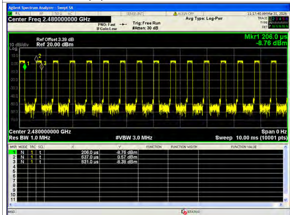
Duty Cycle NVNT BLE 2M 2480MHz Ant2
