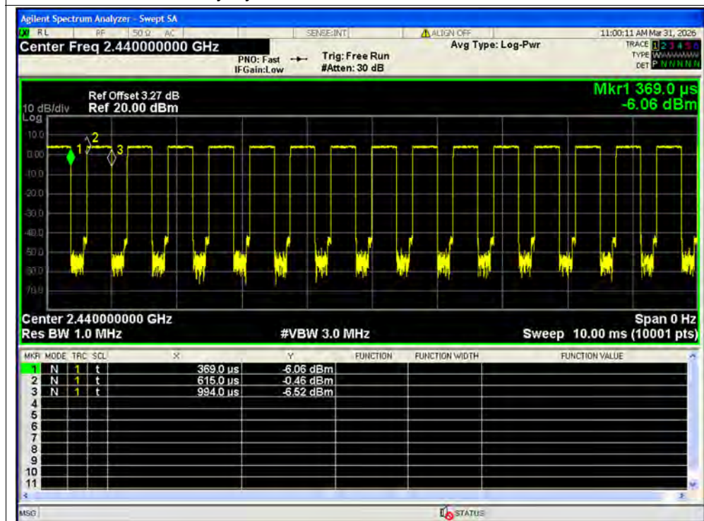
Duty Cycle NVNT BLE 1M 2440MHz Ant2
