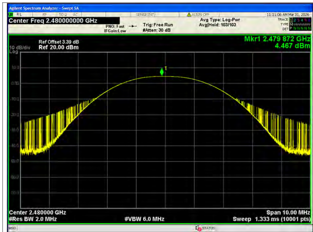
Peak Power NVNT BLE 1M 2480MHz Ant2
