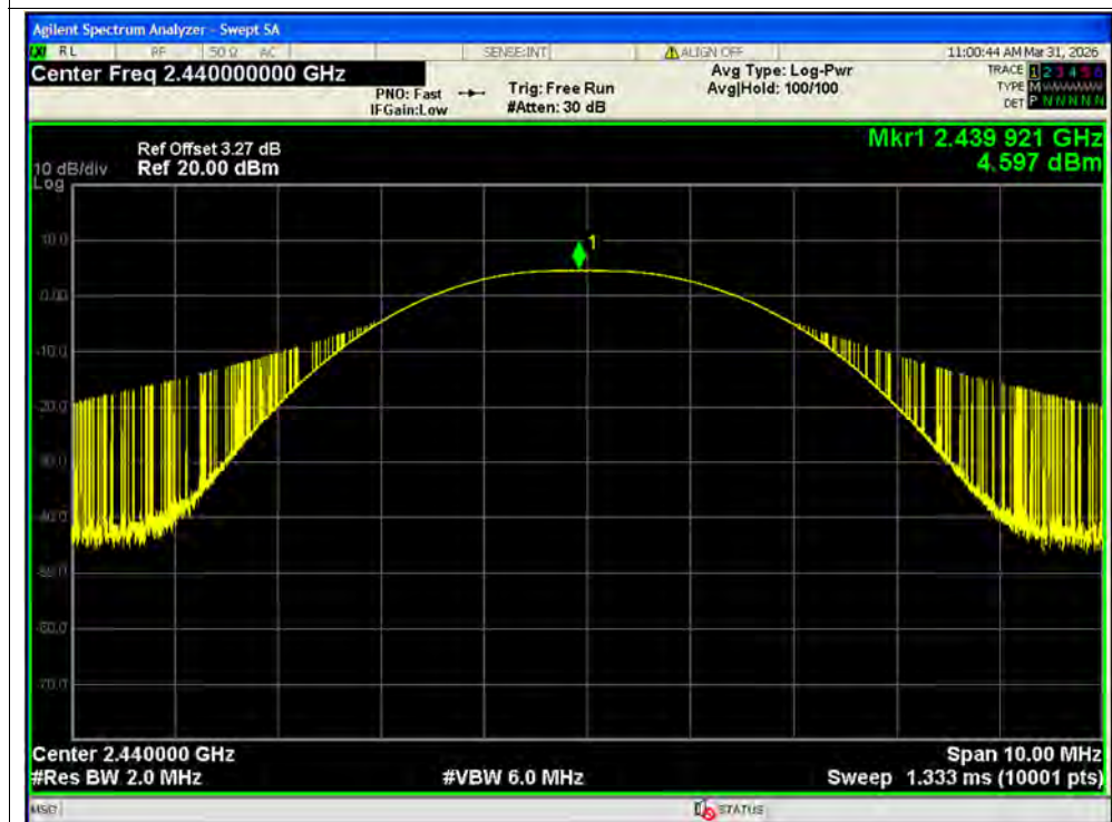
Peak Power NVNT BLE 1M 2440MHz Ant2
