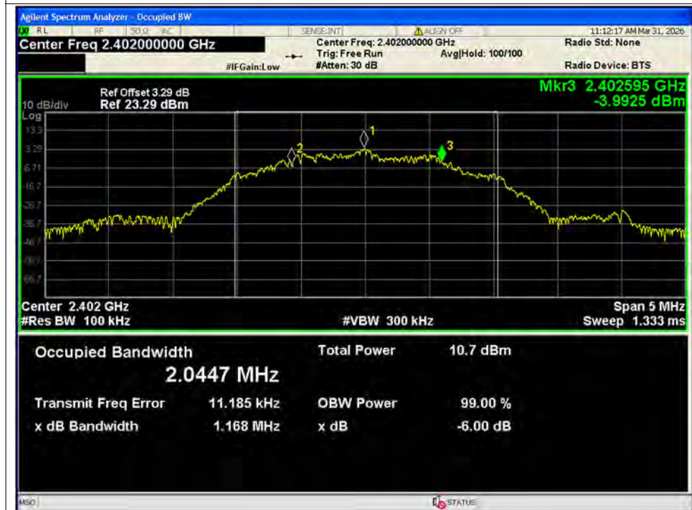
-6dB Bandwidth NVNT BLE 2M 2402MHz Ant2
