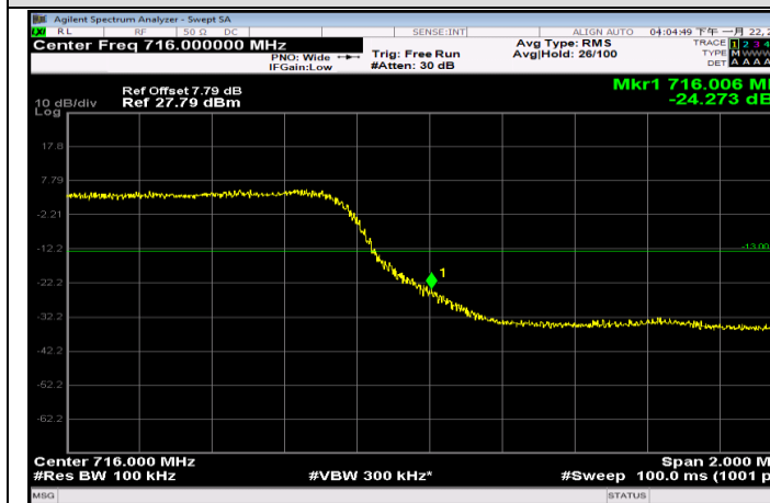
HCH_QPSK_25RB#0
