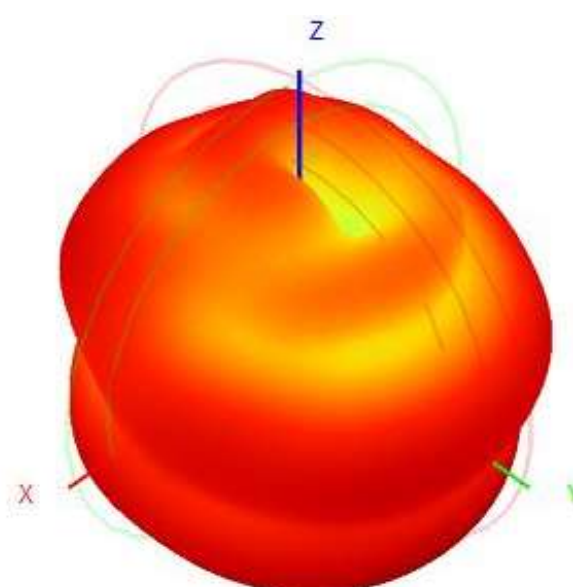
1930MHz
