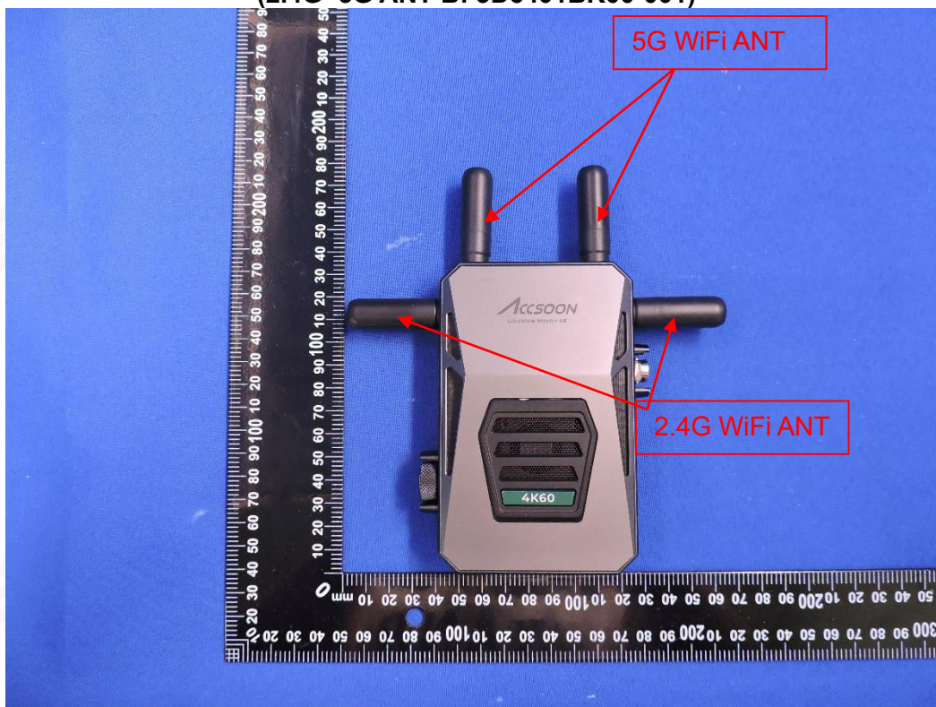
Photo 2 (2.4G+5G ANT B: 3D5401BK00-001)
