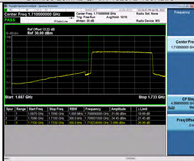
Band66-20MHz-QPSK-132572-1RB#99
