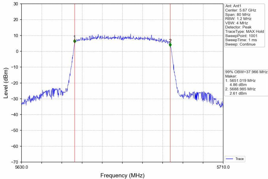
802.11ax(HEW40)_HCH_5670MHz_RU484_Left_Ant1_NTNV
