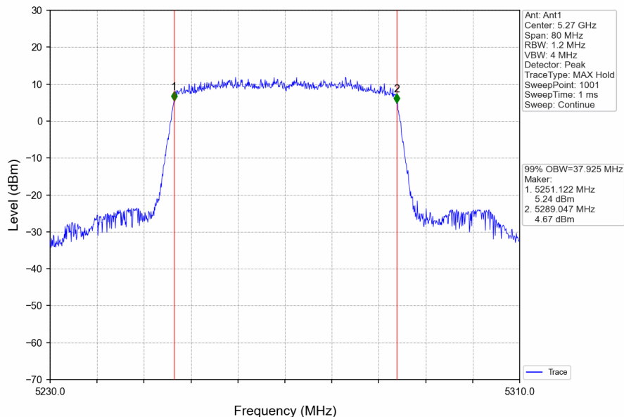
802.11ax(HEW40)_LCH_5270MHz_RU484_Left_Ant1_NTNV
