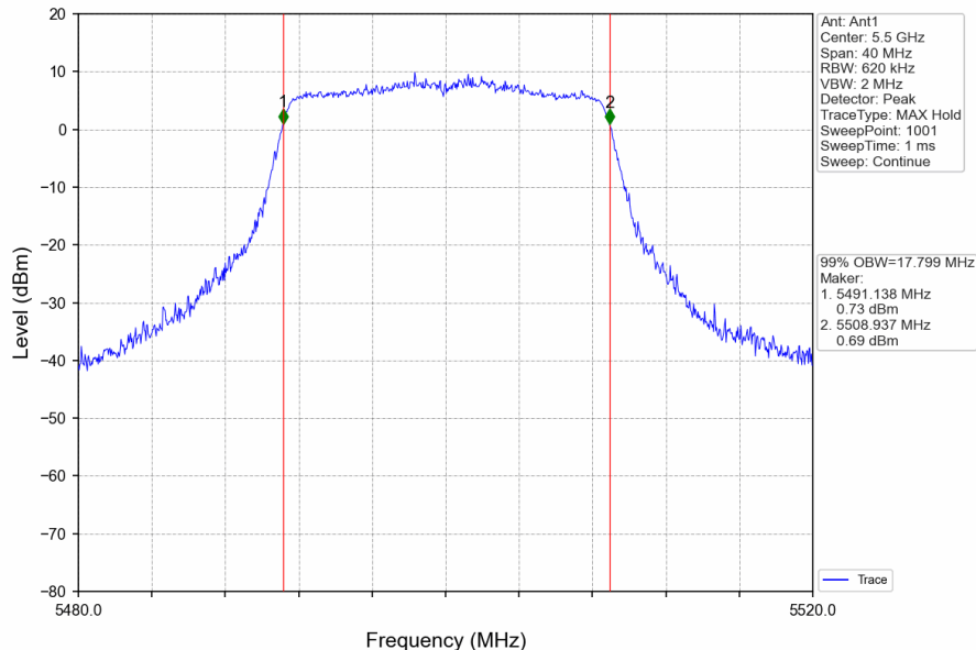
802.11ac(VHT20)_LCH_5500MHz_Ant1_NTNV
