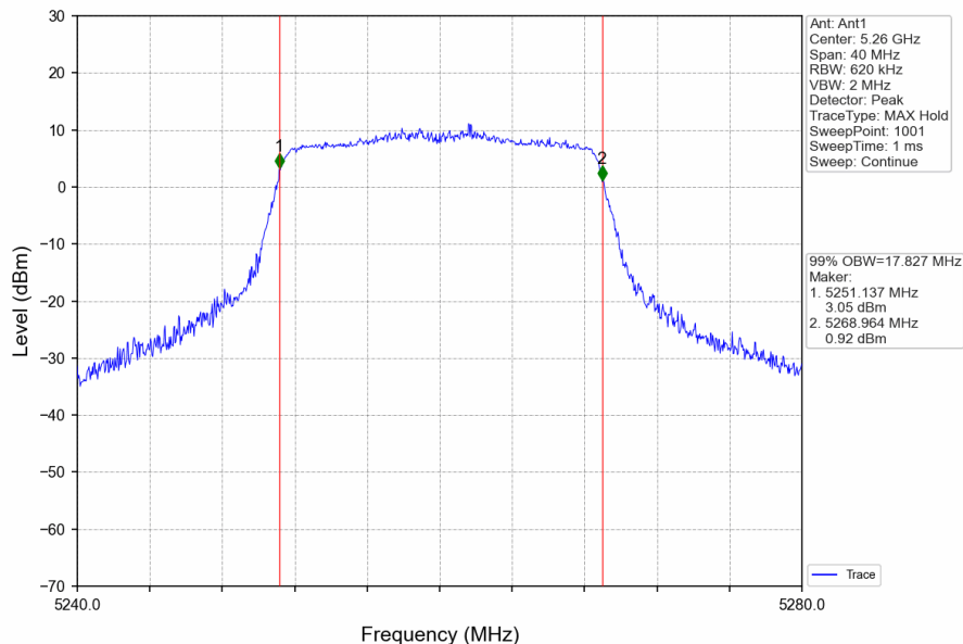
802.11n(HT20)_LCH_5260MHz_Ant1_NTNV
