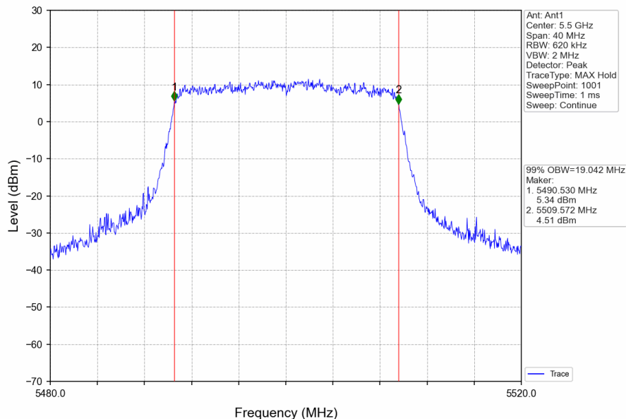
802.11ax(HEW20)_LCH_5500MHz_RU242_Left_Ant1_NTNV
