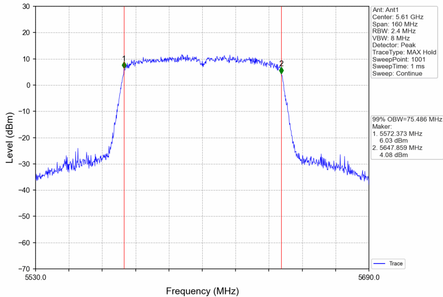
802.11ac(VHT80)_HCH_5610MHz_Ant1_NTNV
