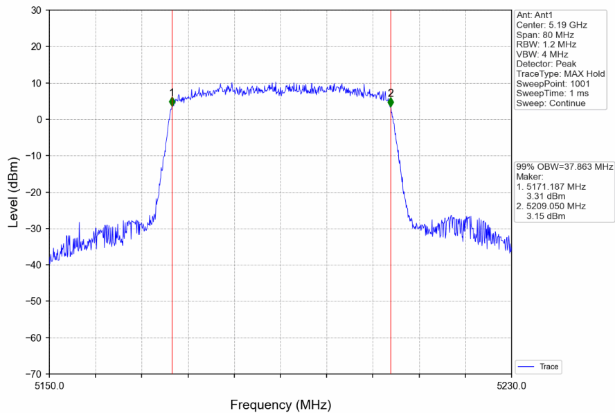
802.11ax(HEW40)_LCH_5190MHz_RU484_Left_Ant1_NTNV
