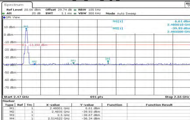
BLE 1M Ant1 High 2480
