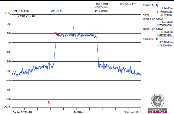
802.11ac(VHT80)_Chain3 / CH155
