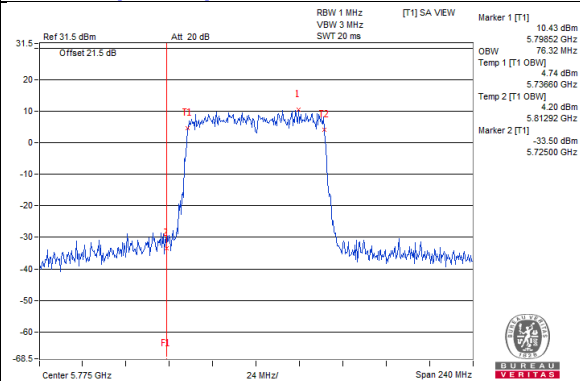
802.11ac(VHT80)_Chain2 / CH155
