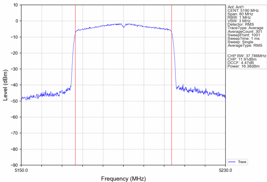
802.11ax(HEW40) LCH 5190MHz RU484 Left Ant1 NTN
