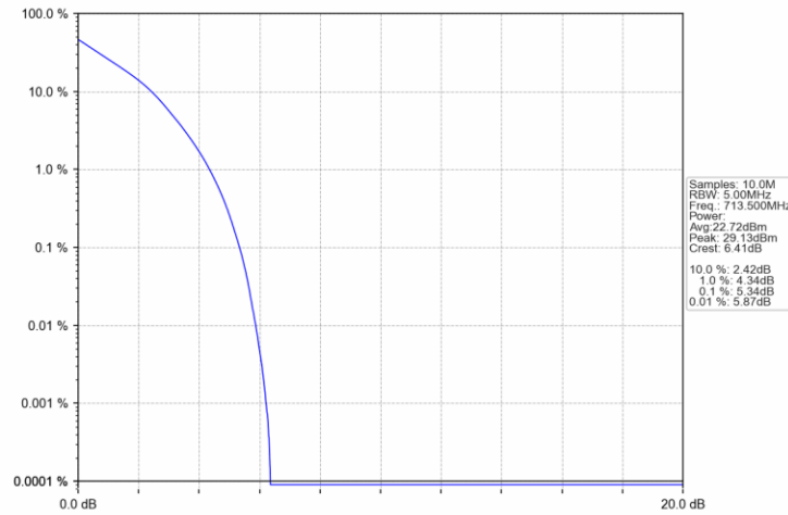
Band17 5MHz QPSK HCH 713.5MHz RB 25 0 NTNV
