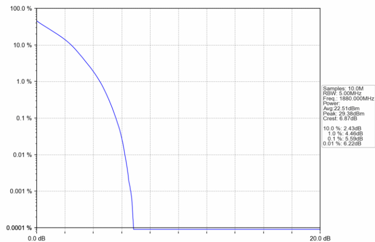
Band2_5MHz_QPSK_MCH_1880MHz_RB_25_0 NTN
