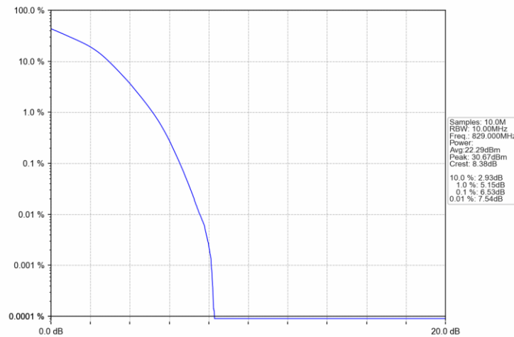
Band5 10MHz 16QAM LCH 829MHz RB 50 0 NTNV
